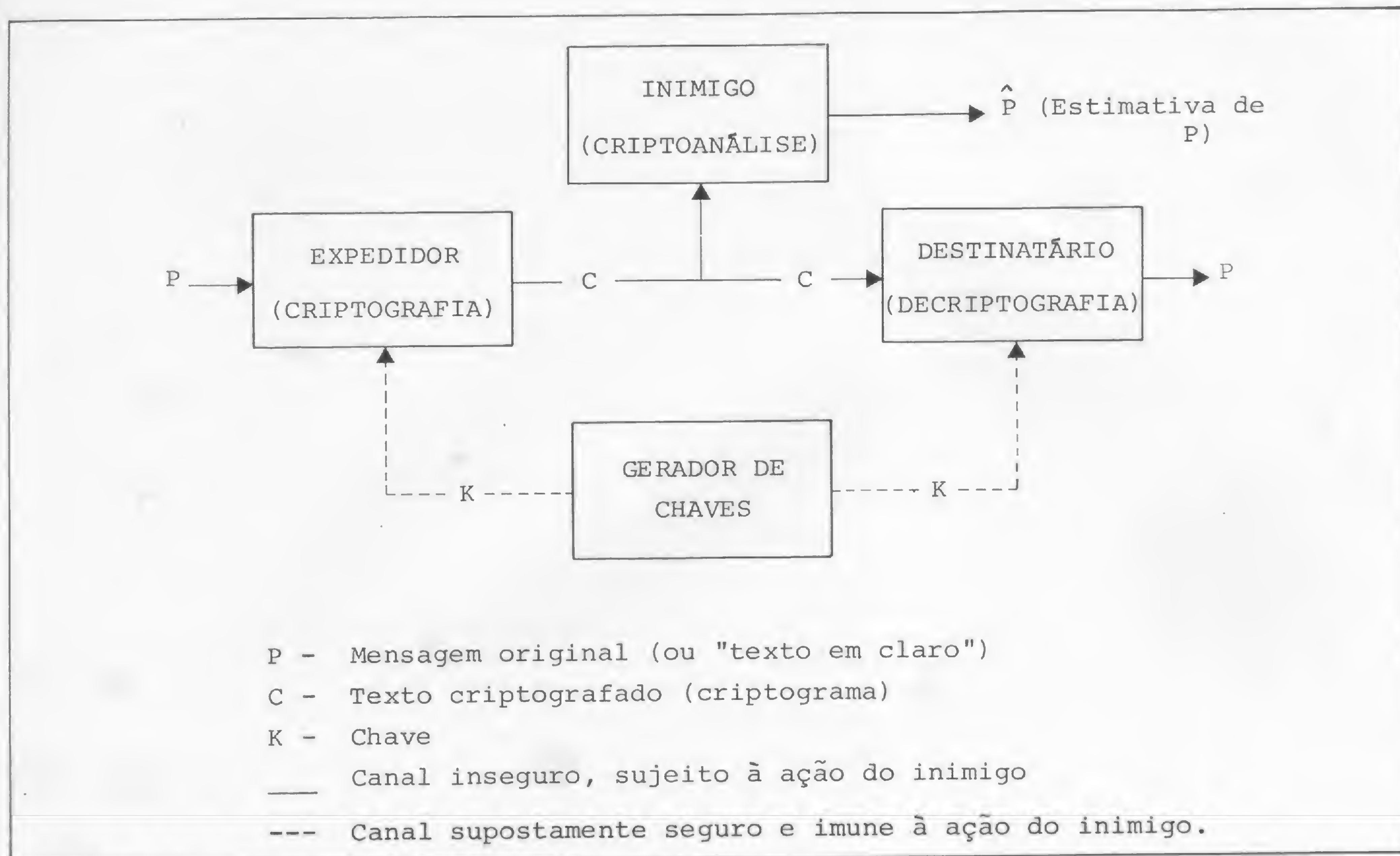
Figura 1 - Esquema do fluxo de informações em um sistema criptográfico convencional/simétrico
